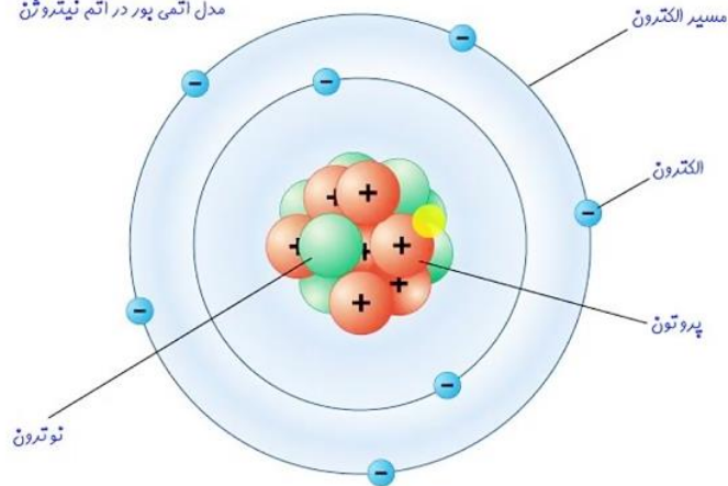
مدل اتمی بور در اتم نیترژن
